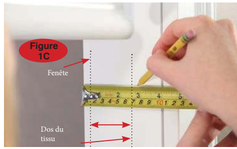
1C Mesurer de la fenêtre jusqu'au dos du tissu en faisant une marque au crayon à trois endroits différents (en haut, au milieu et en bas). Faire une ligne perpendiculaire qui touche les marques et aligner la base Miracle Fit avec cette ligne perpendiculaire.
